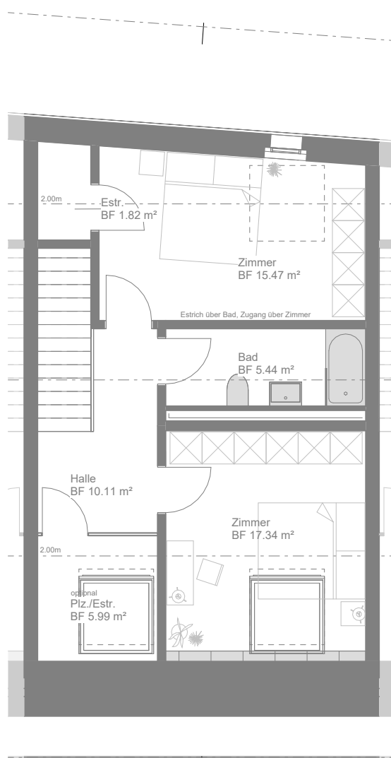
Dachgeschoss
